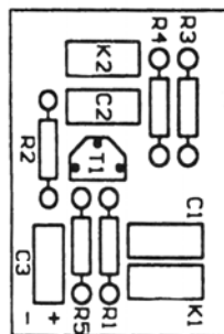
Η τοποθέτηση των υλικών
